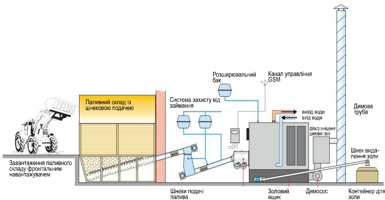
Рис. 3.1.5. Основні елементи котельні на біомасі (деревна тріска).
