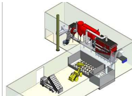
а) компонування котла та паливного складу
