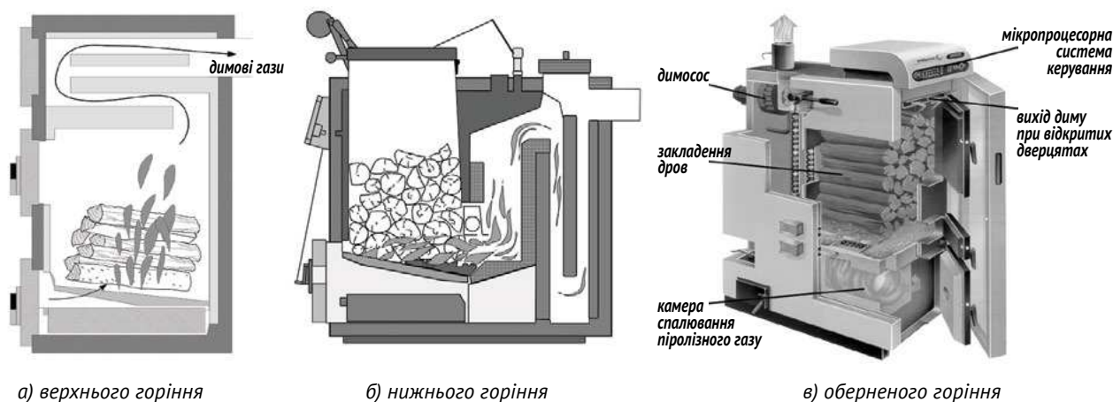
Рис. 3.1.2. Конструкції котлів на дровах.
